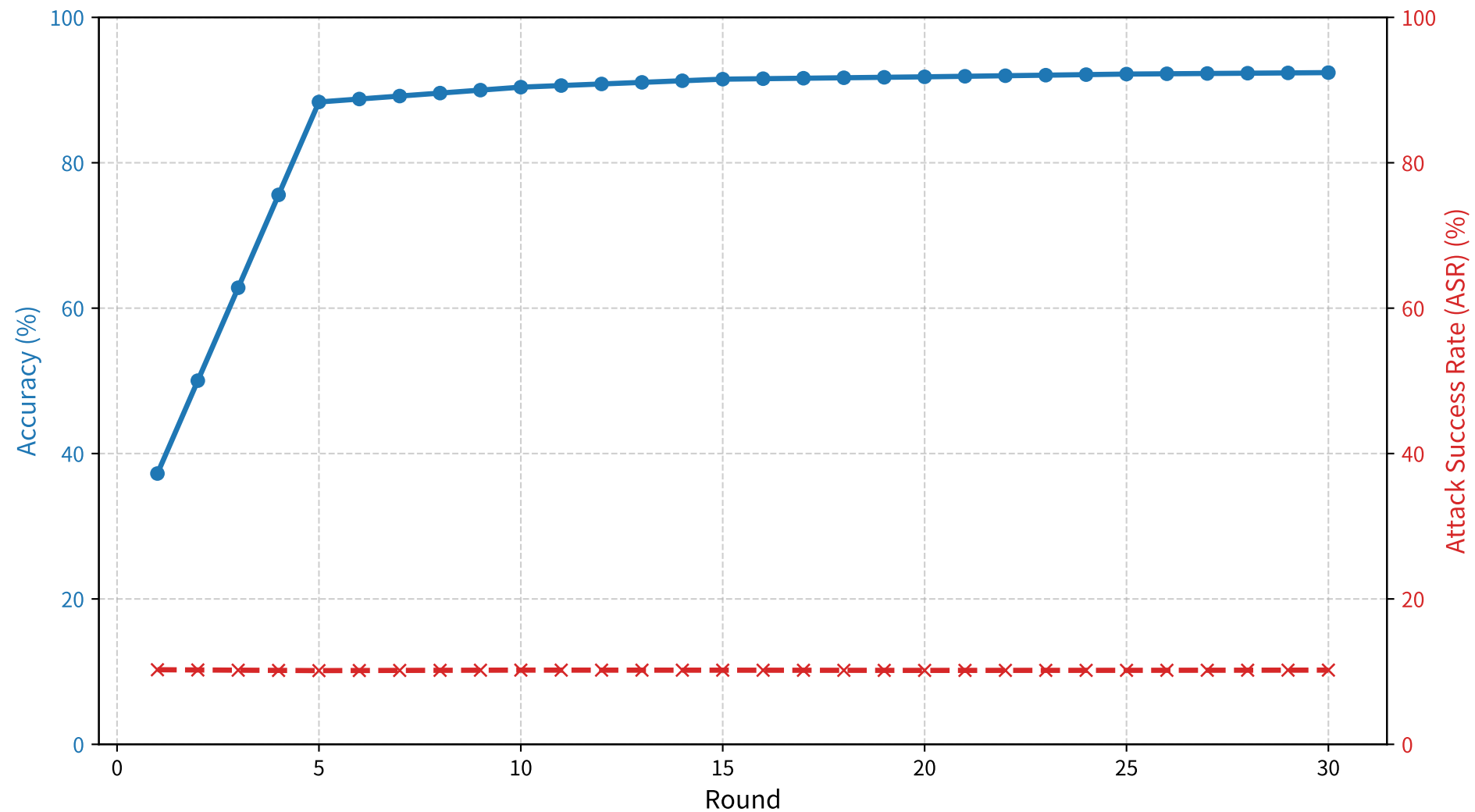
图 3：30轮联邦收敛性与后门 ASR 防范压制能力评估
